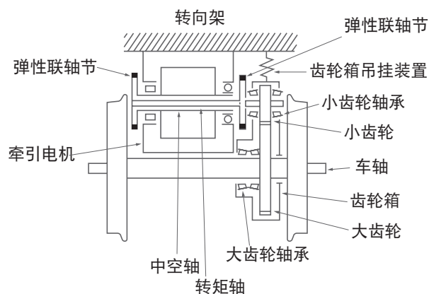
图 3-2 中空轴平行万向节驱动方式
