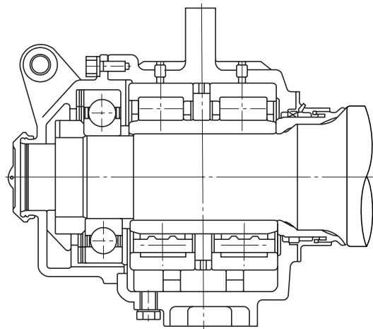
图 1-12 使用可承受轴向负荷的深沟球轴承及盘状垫圈的轴箱
