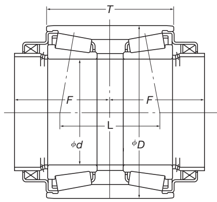
英制系列内置式 RCT
