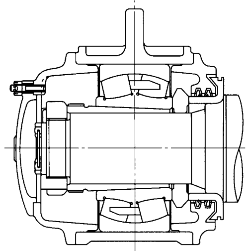
图 1-5 带拆卸套调心滚子轴承
