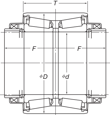
接触式密封型（内置式）
