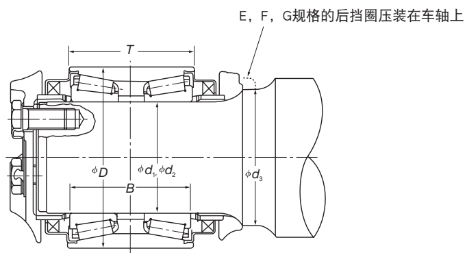
使用前端盖和非覆盖式后挡圈的 RCT (J-360 系列)
