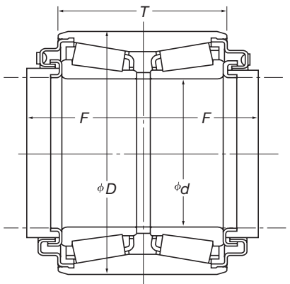
迷宫式密封型（内置式）
