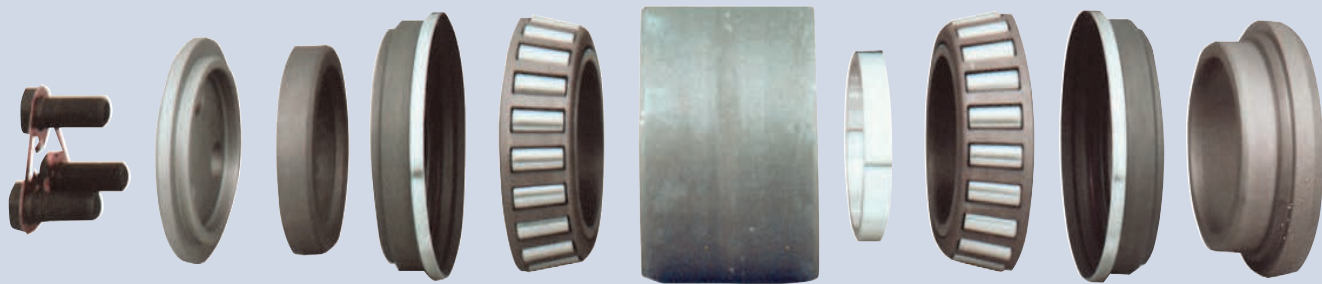
图 1-1 RCT 轴承 (JT14)
