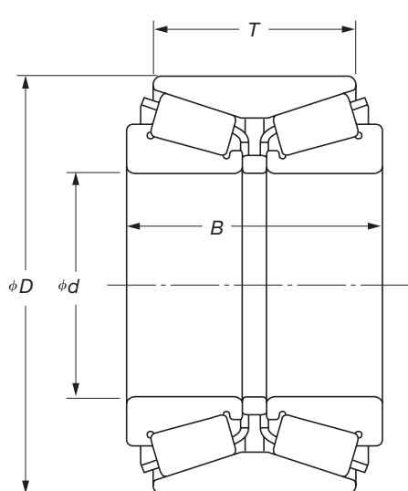
A 型
