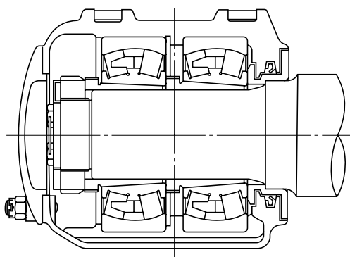
图 1-6 带拆卸套复列调心滚子轴承
