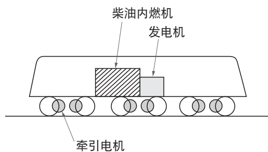
图 3-6 电气式动力传动方式
