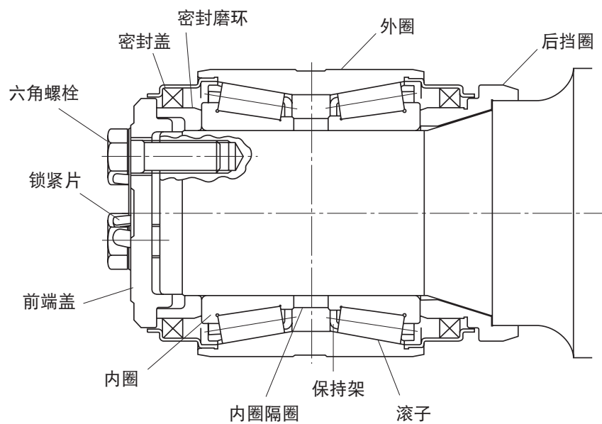
图 1-2 RCT 轴承 (JT14)
