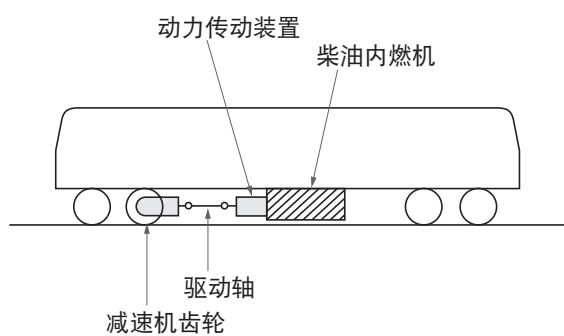
图 3-5 直接或机械式动力传动方式
