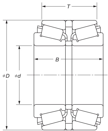
B 型
