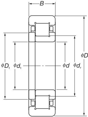
非绝缘轴承
