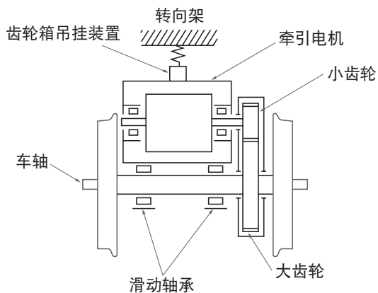
图 3-1 牵引电机吊挂式驱动方式
