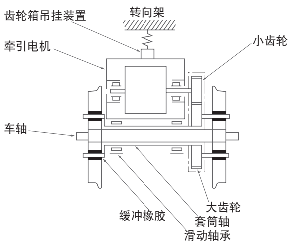
图 3-3 套筒轴式驱动方式
