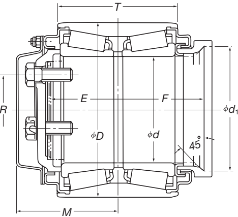
迷宫式密封型（外置式）
