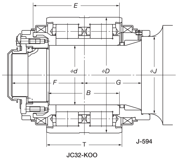
RGC轴承尺寸表
