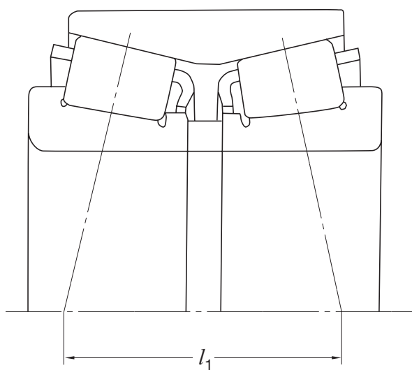
图 1-14 背对背组合
