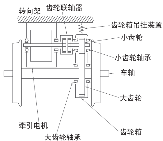
图 3-4 齿轮联轴器式平行万向节驱动方式
