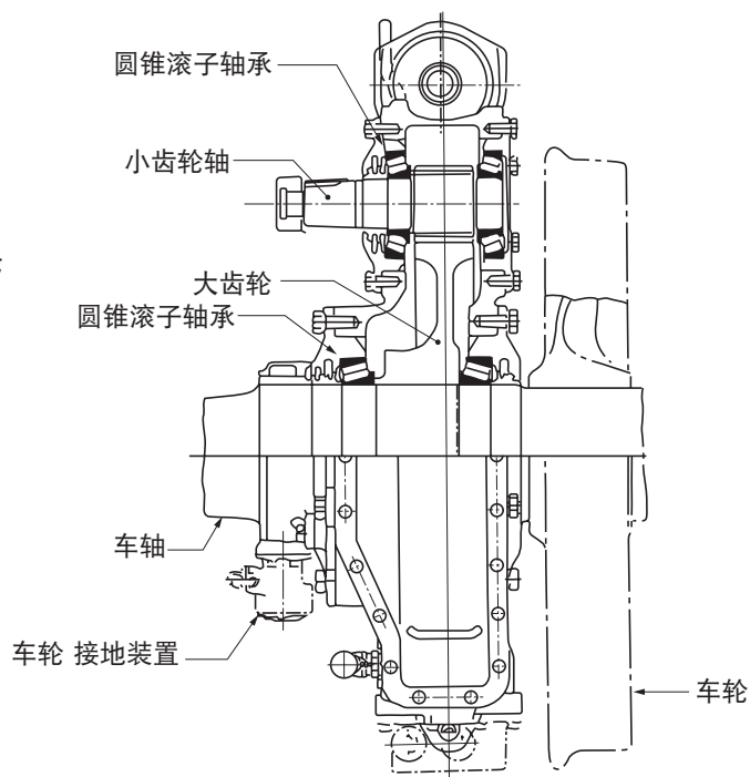
图 3-9 齿轮联轴式平行万向节驱动方式
