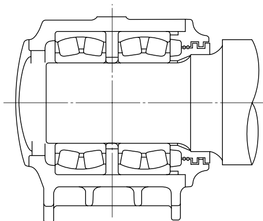
图 1-7 复列调心滚子轴承
