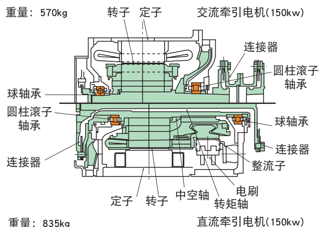
图 2-1 交流牵引电机同直流牵引电机的比较
