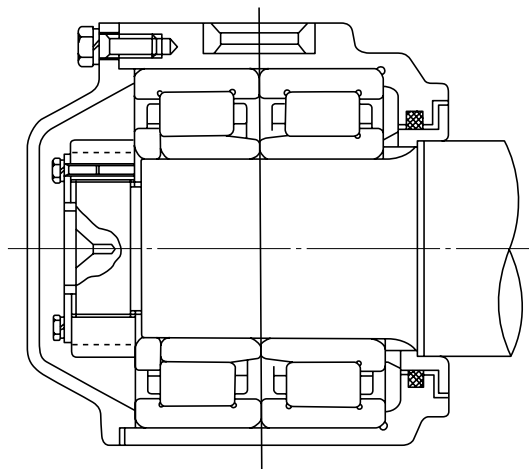
图 1-11 可承受轴向负荷的带挡边复列圆柱滚子轴承 (UIC 标准)
