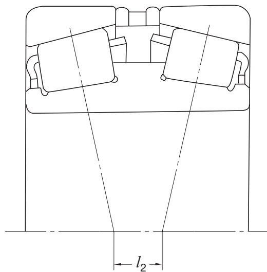
图 1-15 面对面组合
