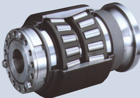
图 1-3 RCT 轴承 (WJT1)
