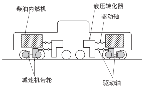
图 3-7 液力传动方式
