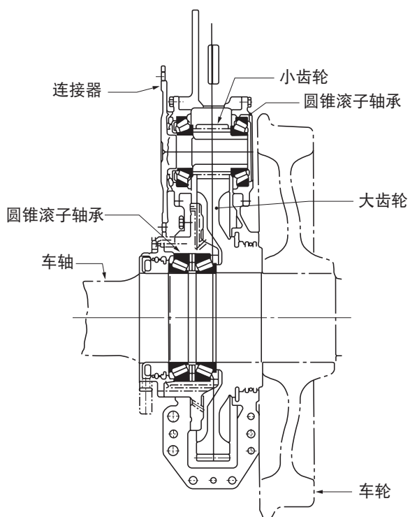
图 3-8 中空轴式平行万向轴驱动装置
